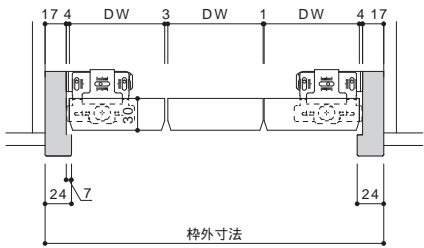
3 枚折戸
