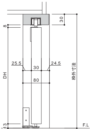
共通縦断面
