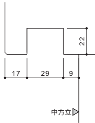
鴨居溝詳細図
