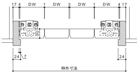
4 枚折戸
