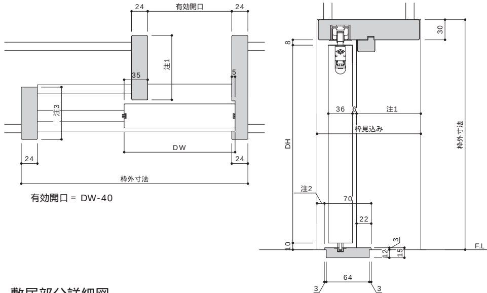
敷居部分詳細図
