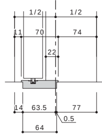
敷居部分詳細図
