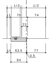
敷居部分詳細図
