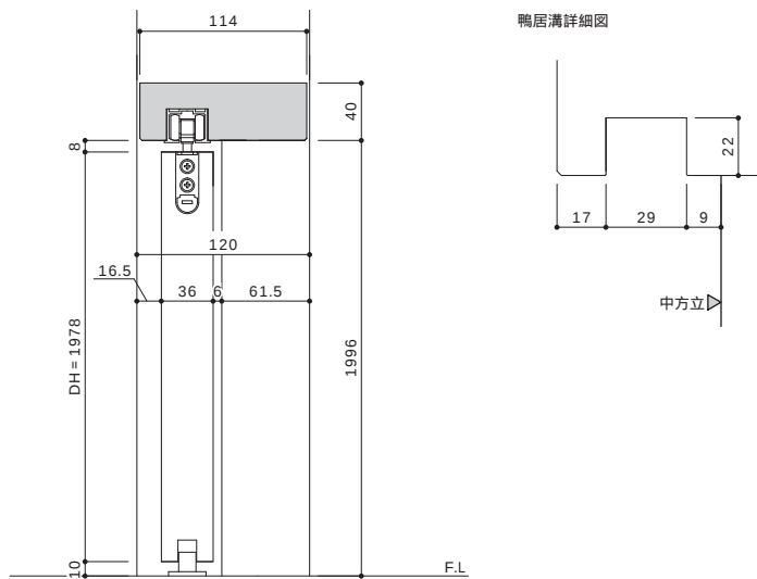
鴨居溝詳細図
