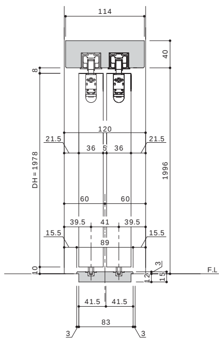
敷居溝詳細図
