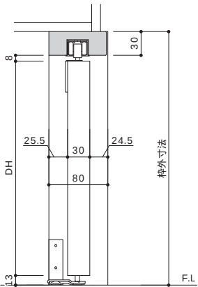
共通縦断面
