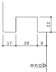
鴨居溝詳細図
