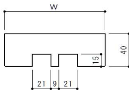
鴨居(L=2,000)
