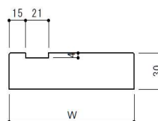
敷居(L=2,000)
